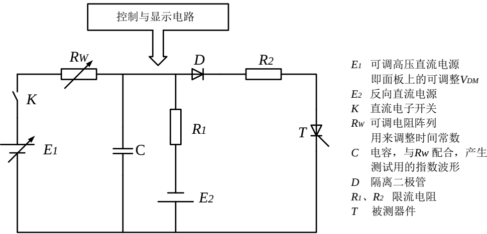
图二、测试原理图
